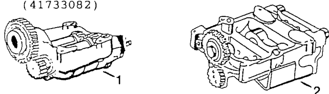
1er modèle (Montage 4 boulons) 2ème modèle (Montage 6 boulons)
